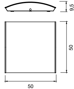
Parete/soffitto - Wall/ceiling 8
