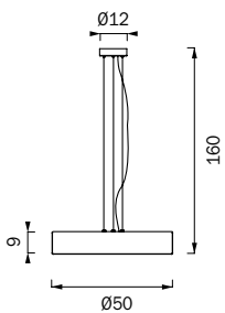
Sospensione - Pendant
