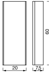
Parete/soffitto - Wall/ceiling 7
