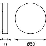
Soffitto/parete - Ceiling/wall
