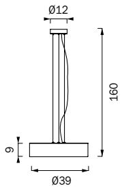
Sospensione - Pendant
