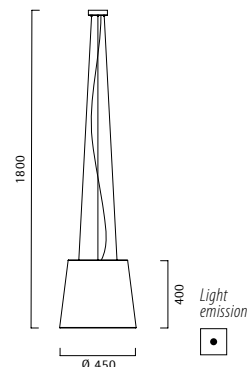
Lampada sospensione - Pendant lamp 004322 Pongè avorio - Ivory pongè E27 2x105W A55 E27 2x100W QT-32 E27 2x21W TC-TSE
