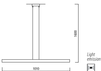
Lampada sospensione - Pendant lamp 000117 Bianco opaco - Matt white LED 6x6W 3.000°K CE V IP30
