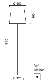
Lampada da terra - Floor lamp 004324 Pongè avorio - Ivory pongè E27 2x105W A55 E27 2x100W QT-32
