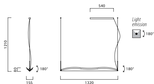
Lampada sospensione - Pendant lamp 012680 Bianco opaco - Matt white G5 1x54W T5 CE V IP20 P
