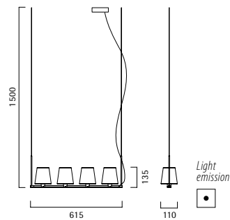
Lampada sospensione - Pendant lamp 004321 Pongè avorio - Ivory pongè G9 4x33W QT-13
