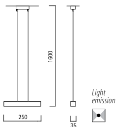
Lampada sospensione - Pendant lamp 000115 Bianco opaco - Matt white LED 2x6W 3.000°K CE V IP30
